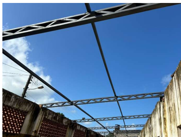
FOTO 6: PINTURA COM ZARCÃO DA ESTRUTURA;
